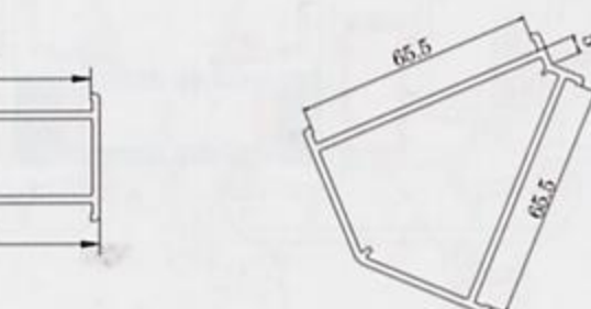
135° Corner-CE135
