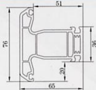
Frame Mullion-GT65N
