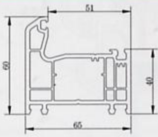
Fixed Frame-GK65
